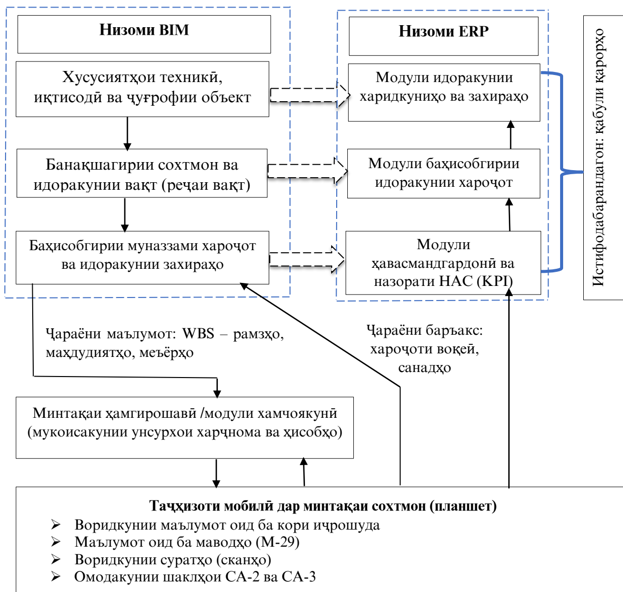
Расми 3.3.1. – Тарҳи ҳамгирокунии низомии BIM ва низомии иттилоотӣ-идоракунии ERP
